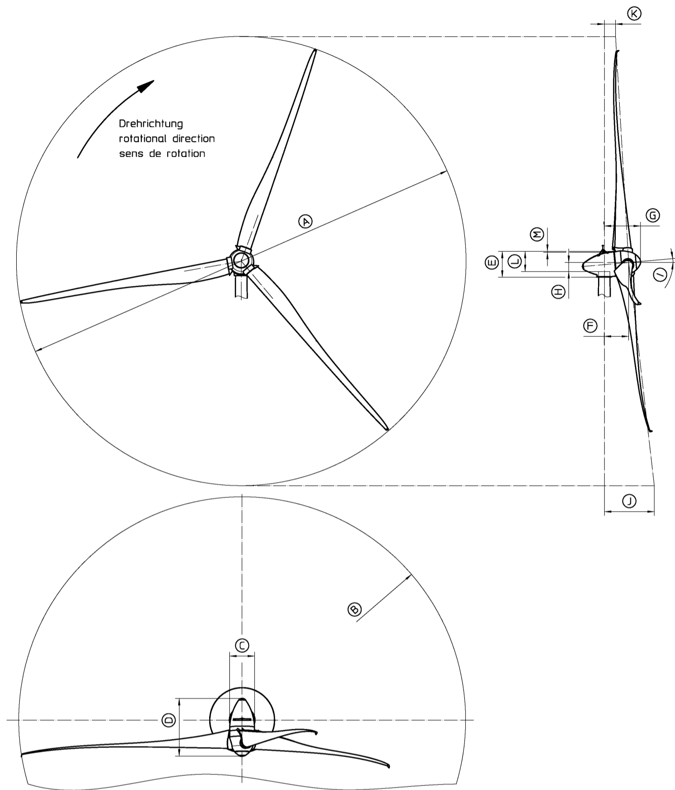
Abb. 1: Schematische Darstellung der Gondel / Schematic diagram of the nacelle / représentation schématique de la nacelle
