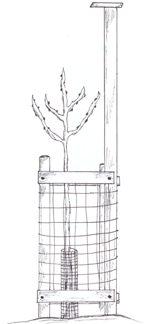
Abb. 3: Anbindung und Verbissschutz wie in Abb. 2, zusätzlich mit integrierter Greifvogelansitzstange.
