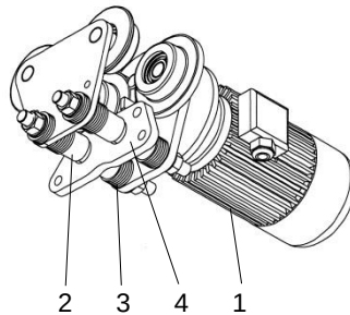
Elektrofahrwerk
