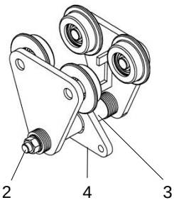
Einbolzenhandfahrwerk
