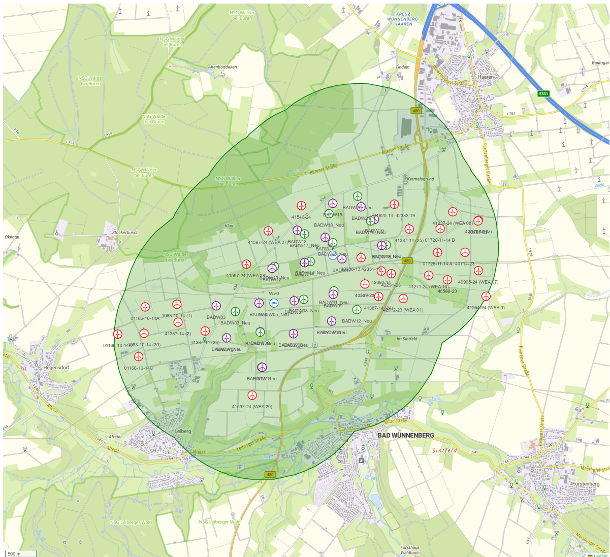
Abbildung 2.1: Lageplan des untersuchten Standortes Bad Wünneberg mit den untersuchten WEA und den Windverteilungspositionen. Zusätzlich sind die 10 D Umgebungen der geplanten WEA dargestellt. [Bun24]
