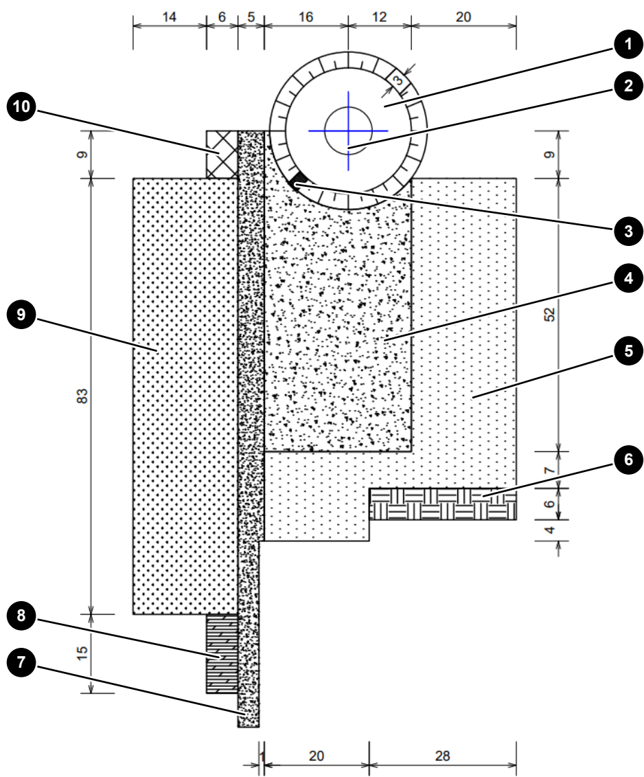
Abb. 15: Alternativer Arbeitsbereich am WEA-Standort, Baumaß (alle Maßangaben in Meter)
