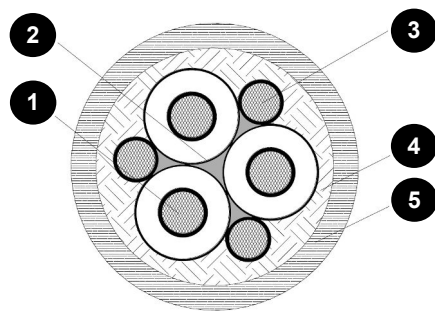
Abb. 4: Kabel Nexans Typ (N)TSCGEHXOEU
