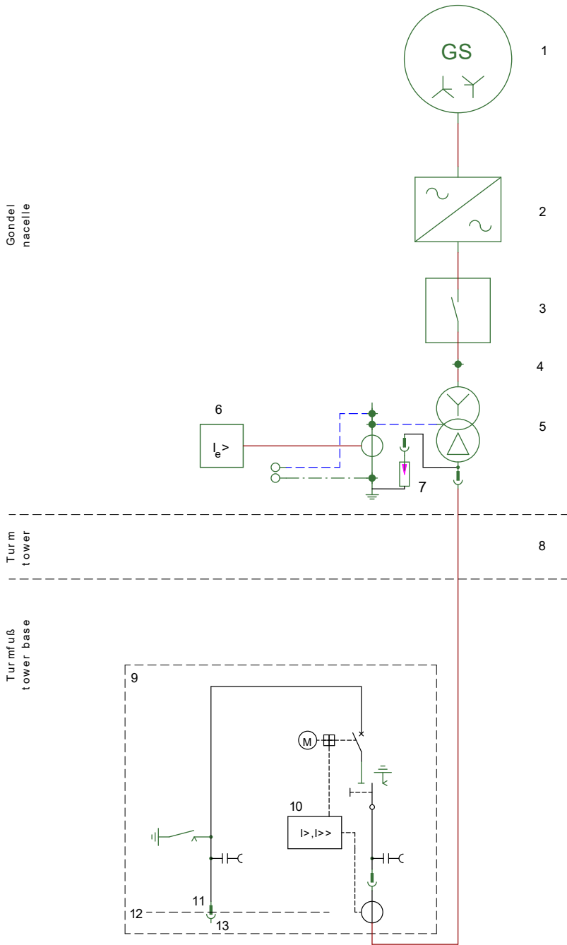
Abb. 1: Prinzipschaltbild – Netzanschlussvariante 6
