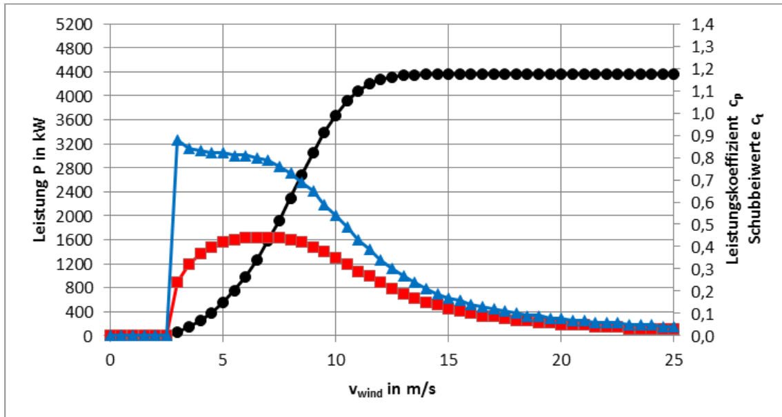
Abb. 1: Leistungs-, c_p - und c_t -Kennlinien E-147 EP5 / 4300 kW Betriebsmodus 0 s
