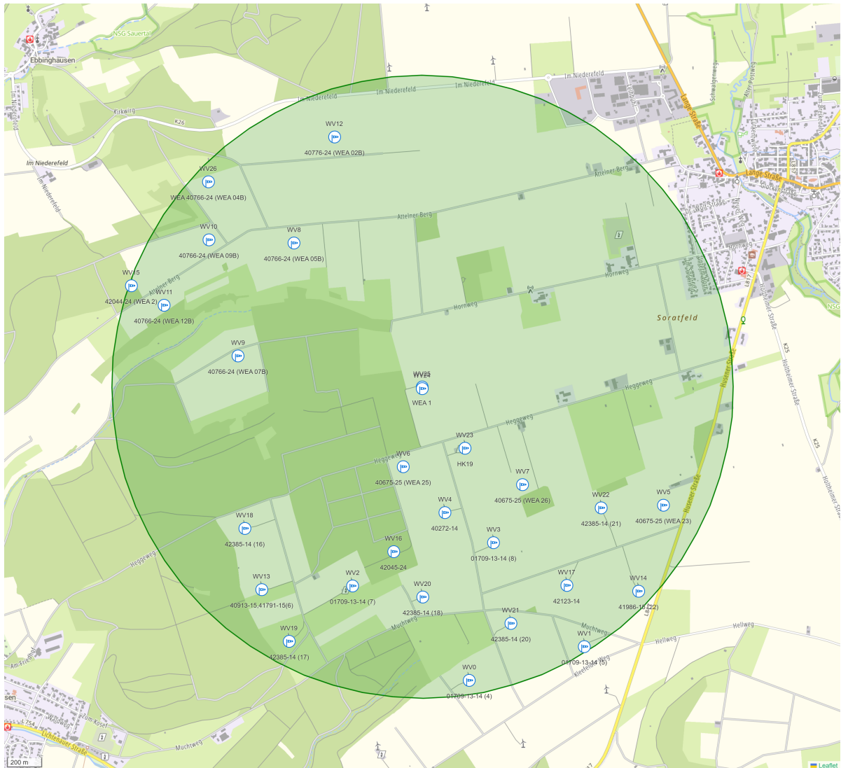
Abbildung 2.1: Lageplan des untersuchten Standortes Lichtenau mit den untersuchten WEA und den Windverteilungspositionen. Zusätzlich sind die 10 D Umgebungen der geplanten WEA dargestellt. [Bun24]
