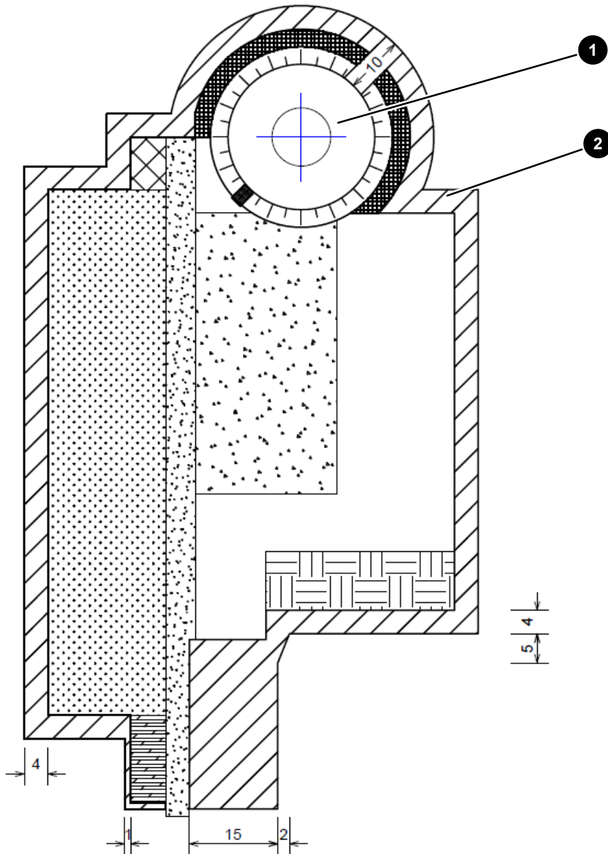
Abb. 16: Alternativer Rodungs- und Sicherheitsbereich, Baumaß (alle Maßangaben in Meter)
