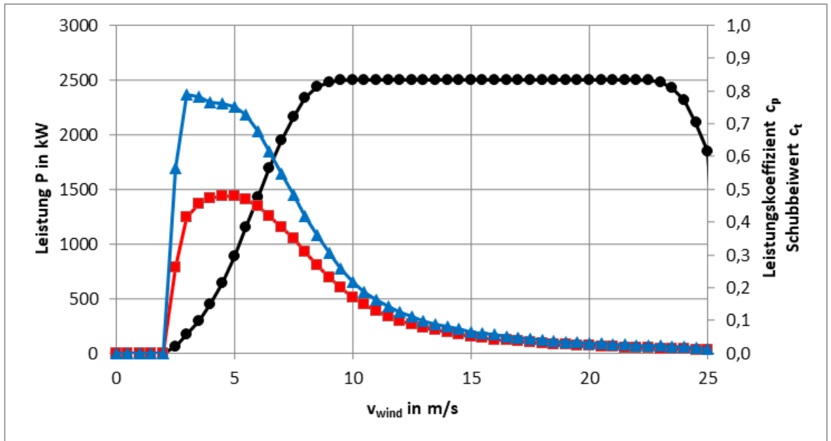
Abb. 1: Leistungs-, c_p - und c_t -Kennlinien E-175 EP5 E2 / 7000 kW Betriebsmodus OM-NR-09-0
