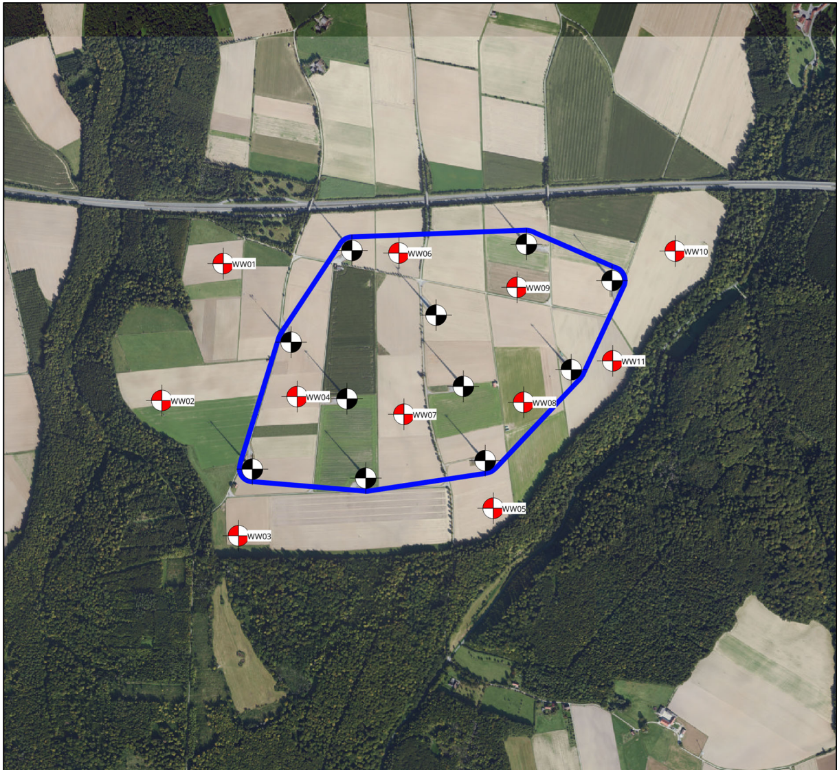
Abbildung 3 Plan des Standortes der WEA WW01 im WP Wewelsburg mit Umgebung
