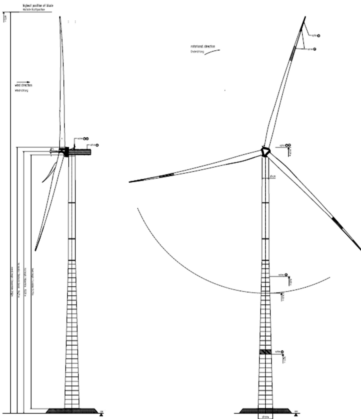
Abbildung 1: Übersichtszeichnung einer Enercon E-175 EP5 mit 162 m Nabenhöhe (Quelle: Enercon)
